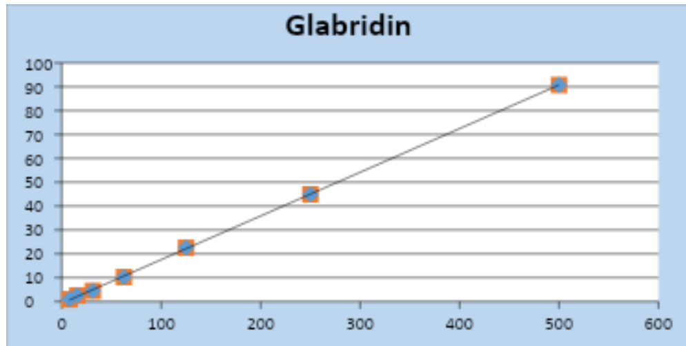
איור 1: עקומת כיול עבור Glabridin
